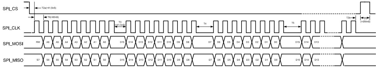
AiP4952C/D SPI 时序格式
