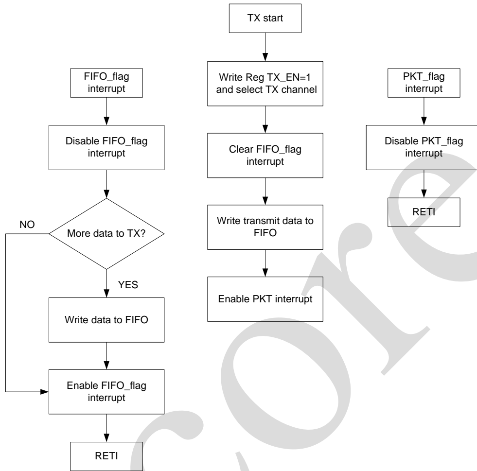
MCU 发送数据包流程图
