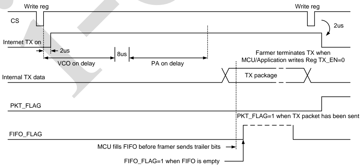
当寄存器 0x01[2:1]=2'b00 时，TX 时序图
