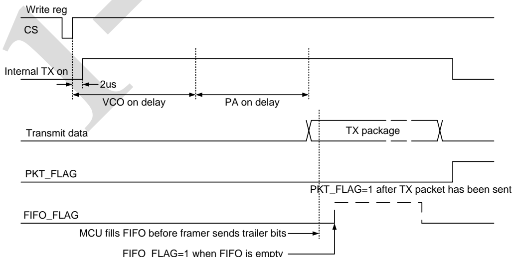
TX 时序图
