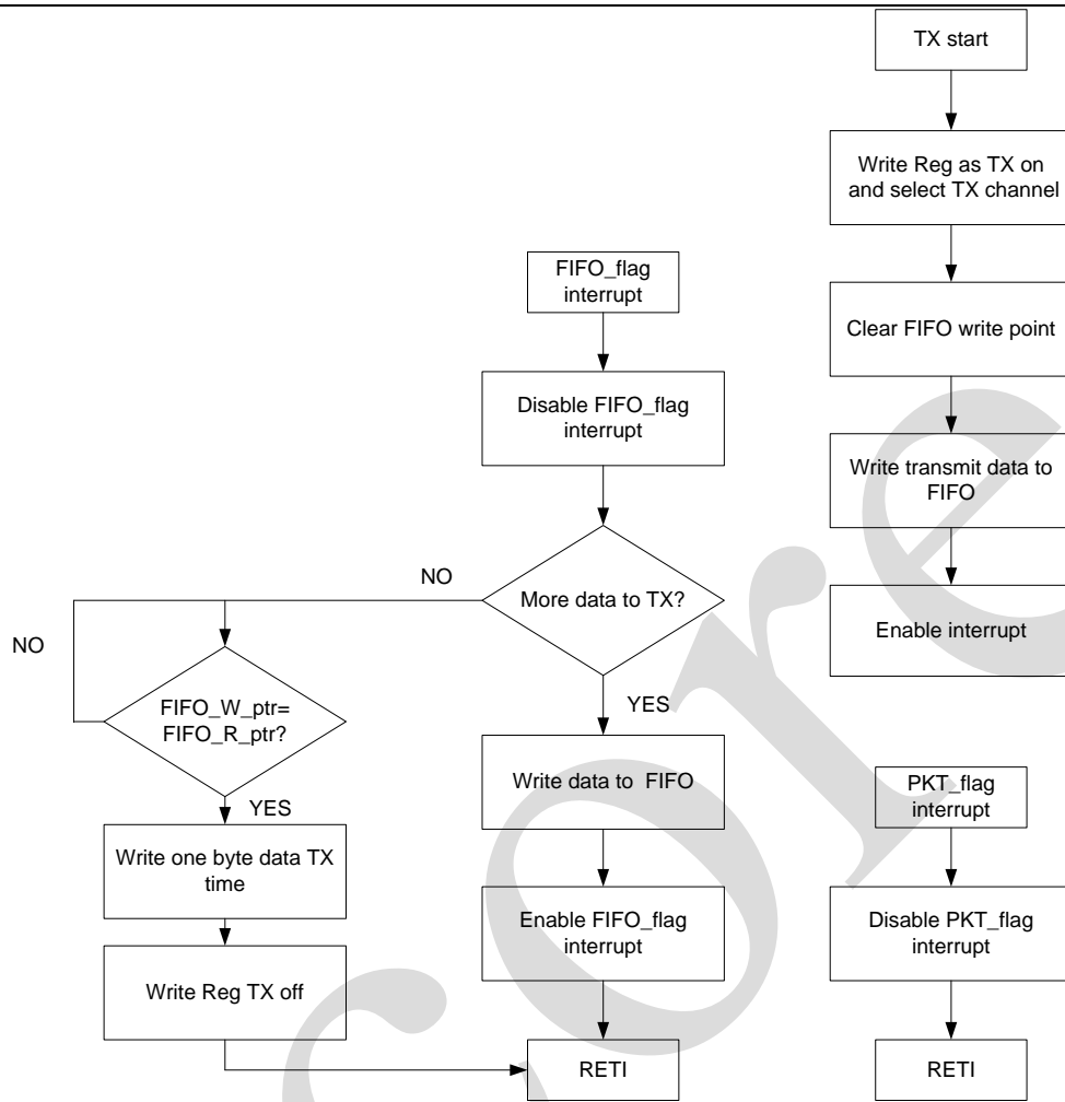
当寄存器 0x01[2:1]=2'b00 时, TX 流程图
