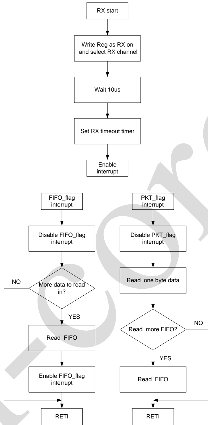
当 Reg0x01[2:1]='b00 or 'b01 时, RX 流程图
