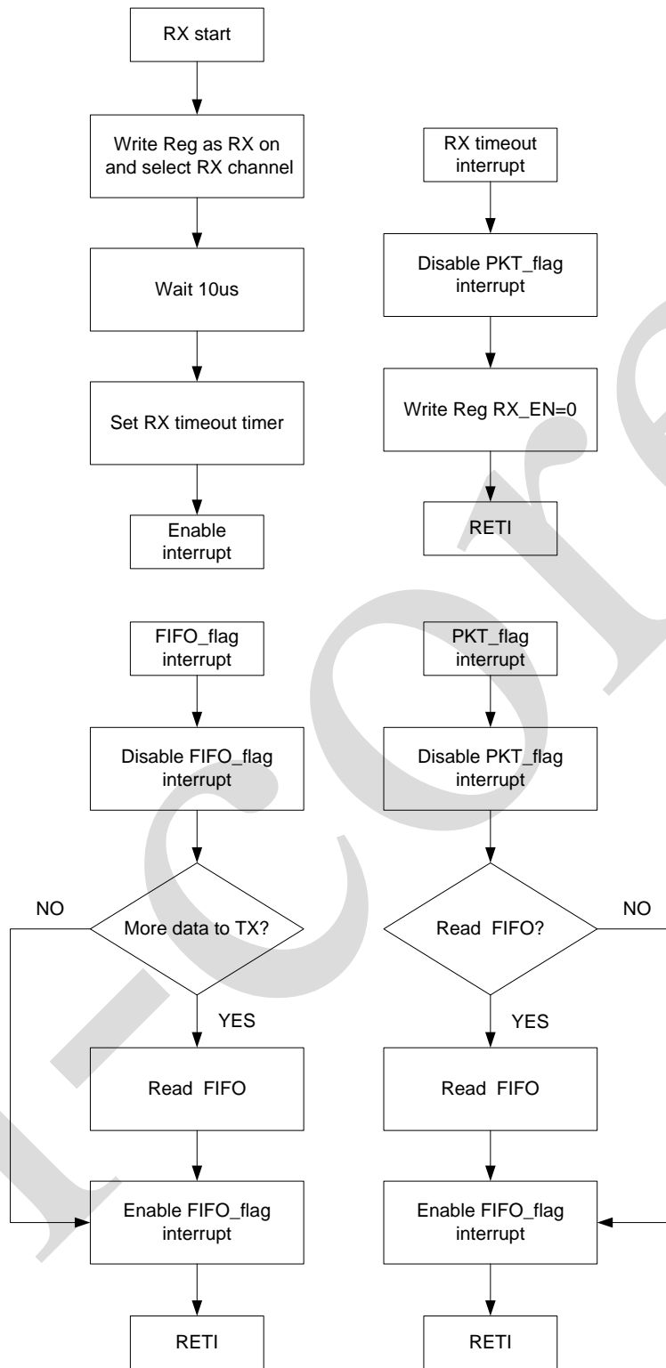
接收流程图
