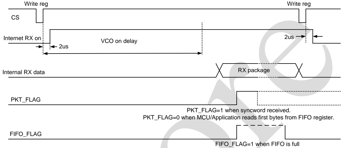
当 Reg0x01[2:1]='b00 or 'b01 时, RX 时序图
