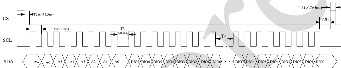
AiP4952A SPI 时序格式
