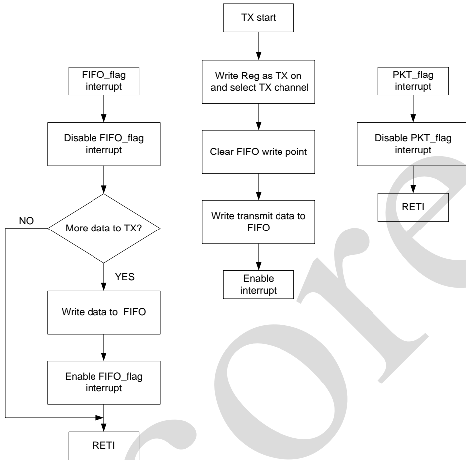
寄存器 0x01[2:1]=2'b01 时发射的流程图
