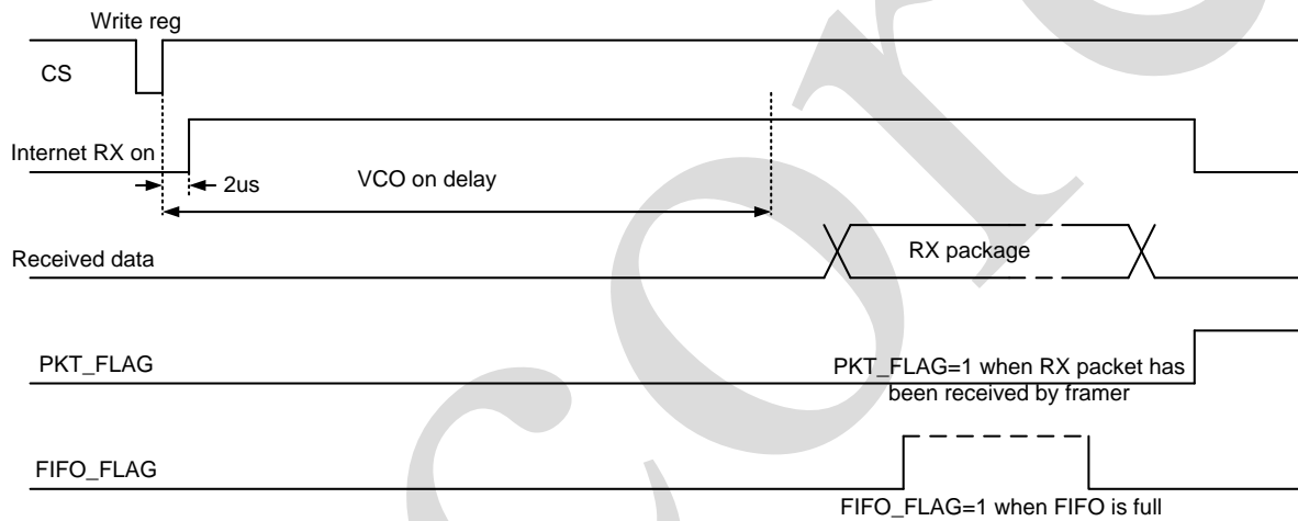
接收时序图
